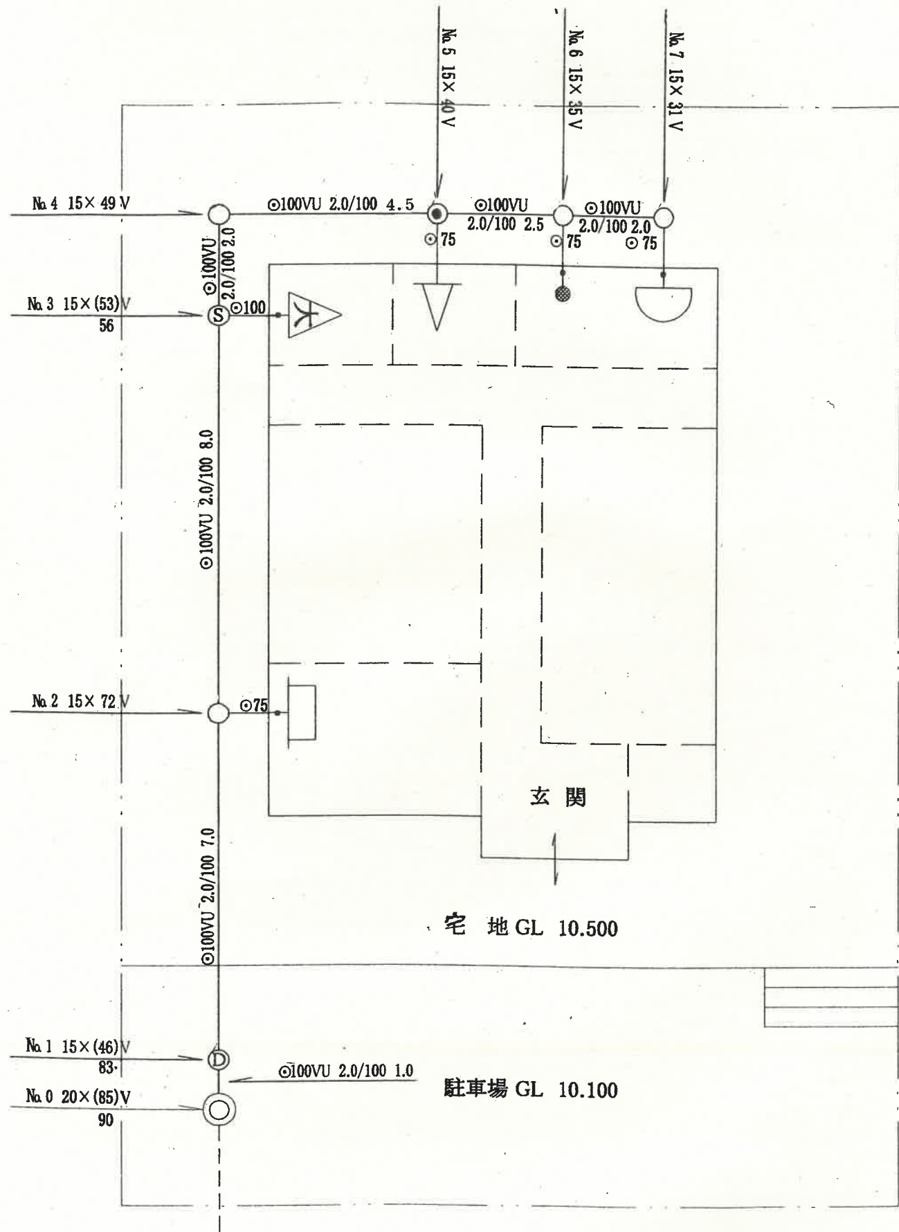
平面図 S=1/100(分流式)
